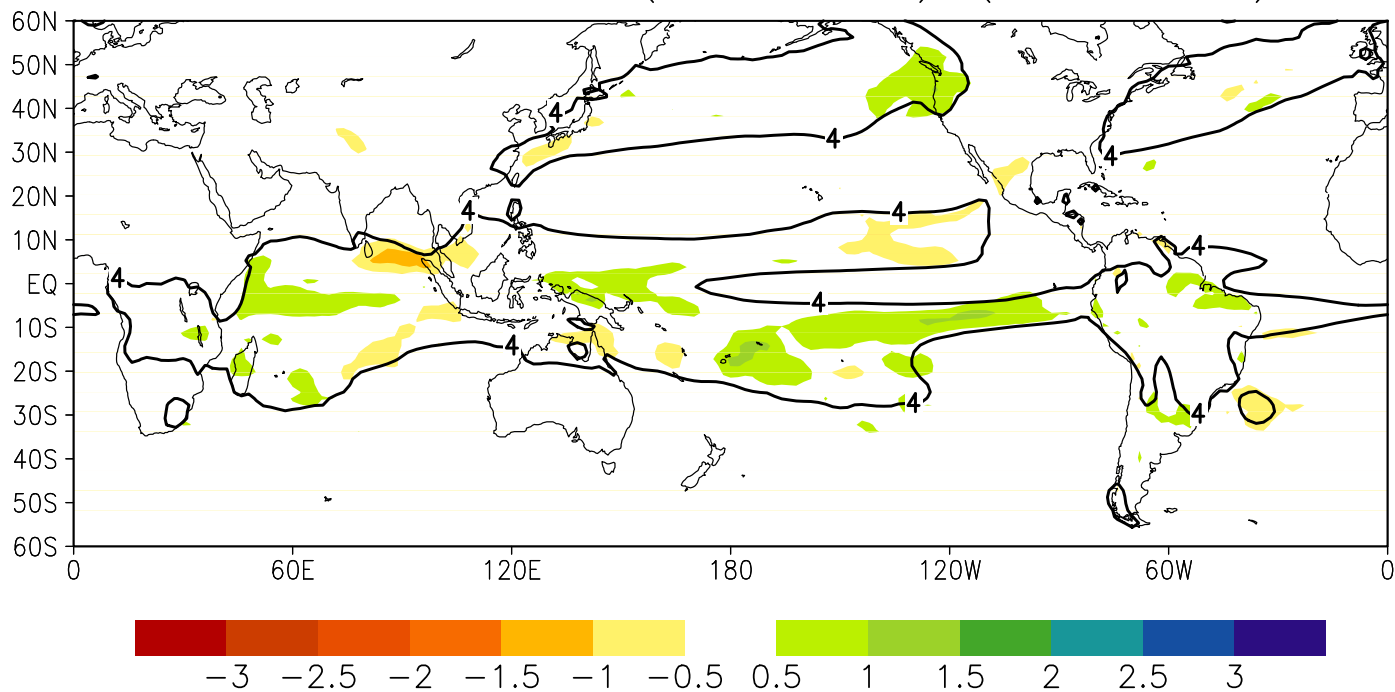
inmcm4 DJF Pa(1976-05) (1850-79)
