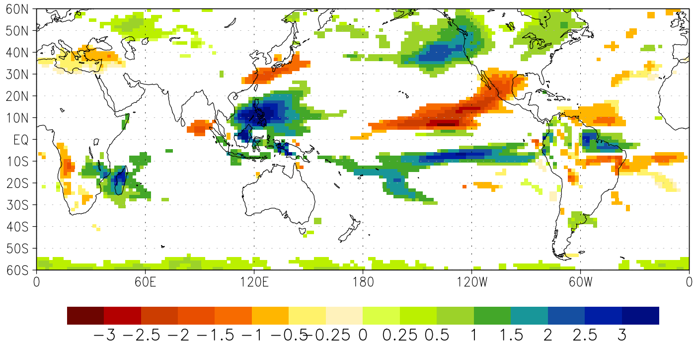
inmcm4 DJF Pra(2085) wrt 1850-79 (95%)
