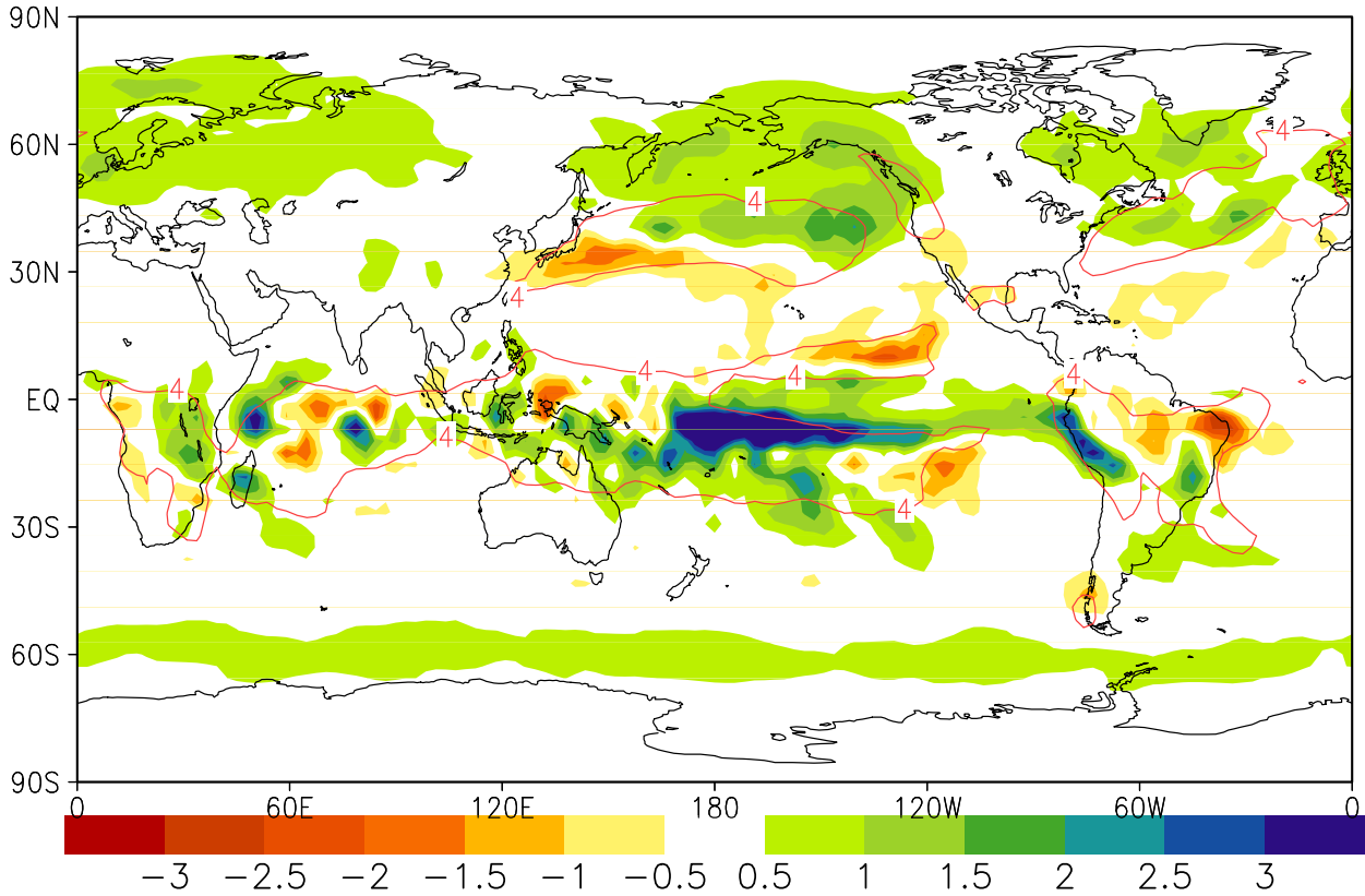
mip5 bcc esmrcp8.5 DJF Prec(2070-99) (1850-79)
