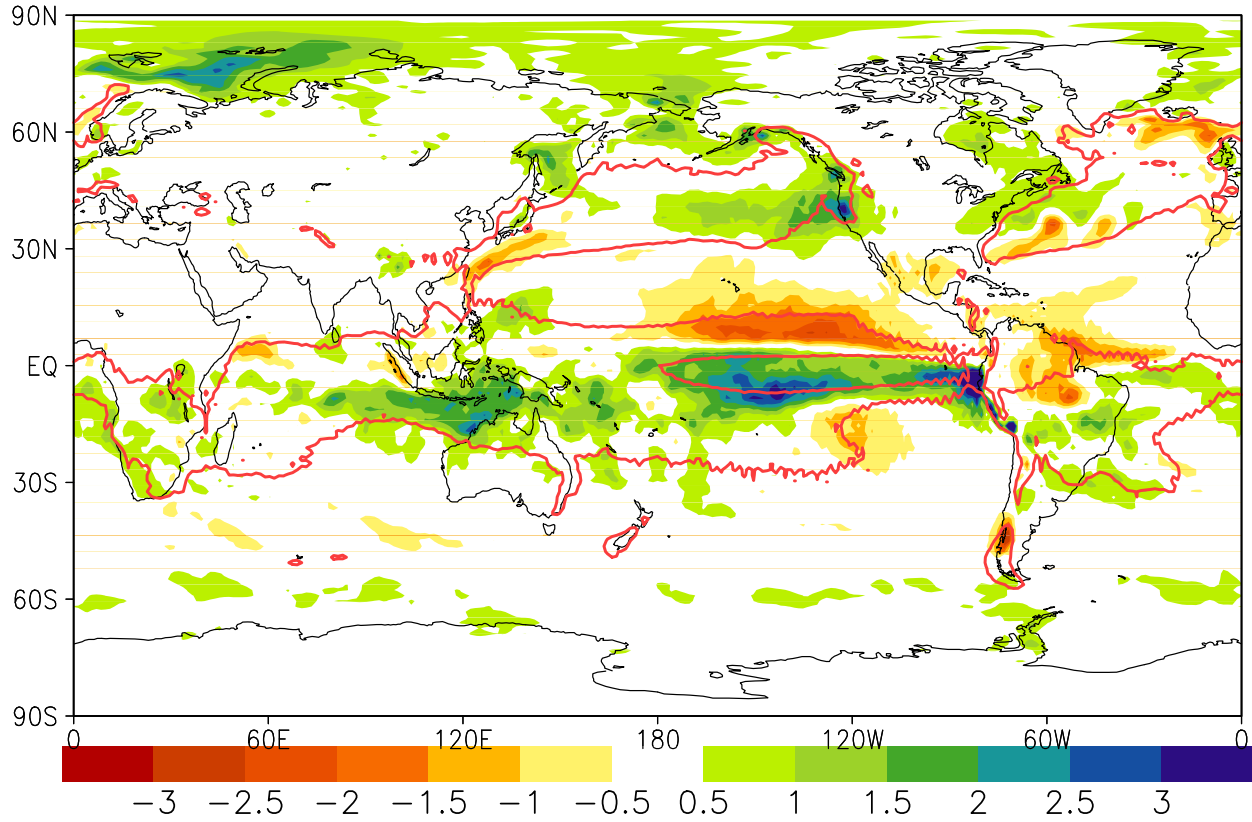
cmip5 cnrm rcp8.5 DJF Prec(2070-99) (1850-79)
