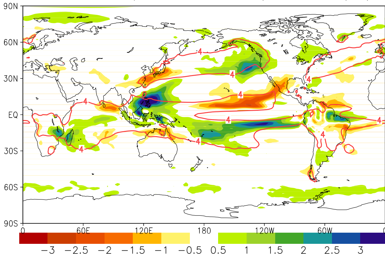
rip5 inmcm esmrcp8.5 DJF Prec(2070-99) (1850-79)
