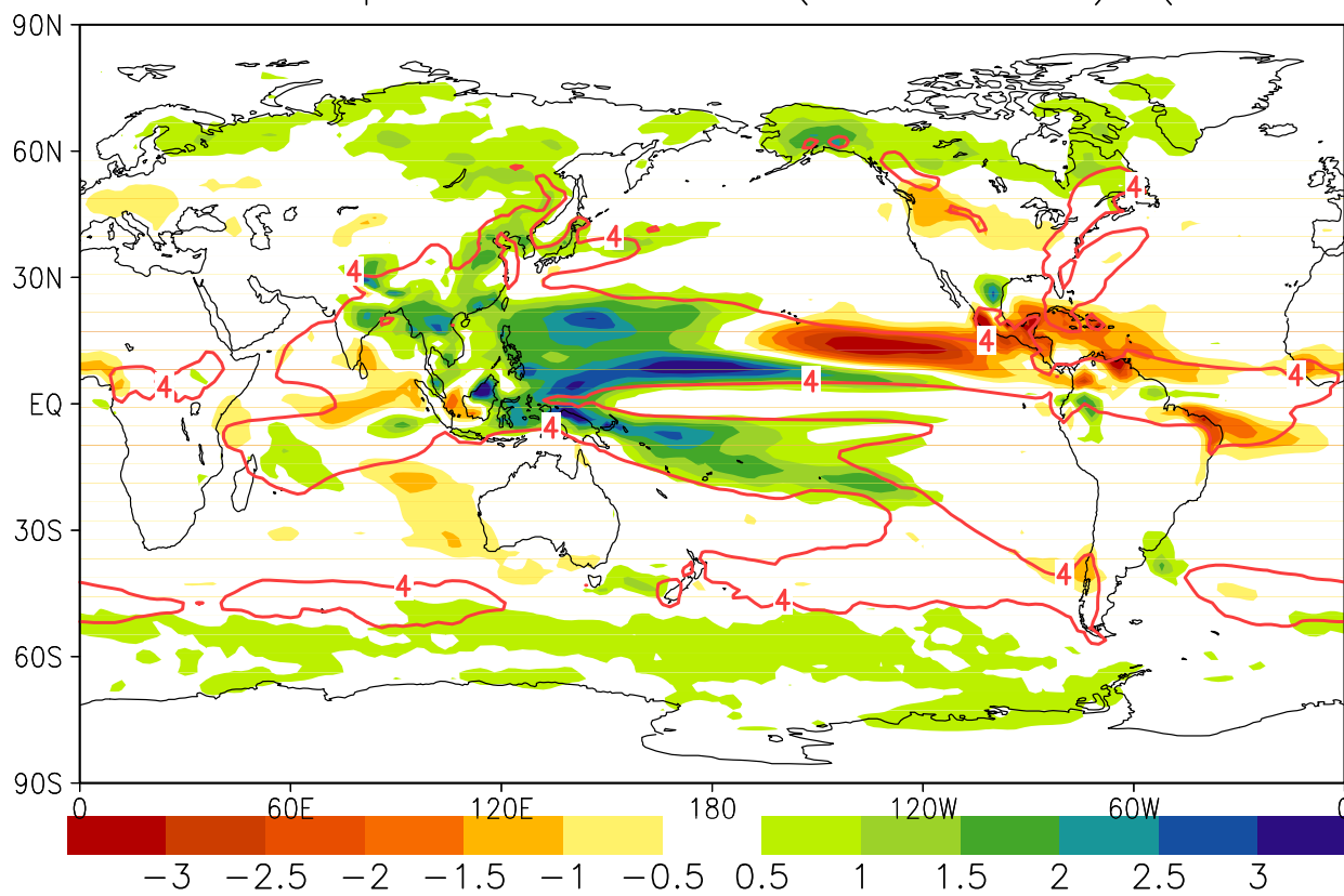
inmcm esmrcp8.5 JJA Prec(2070-99) (1850-79)
