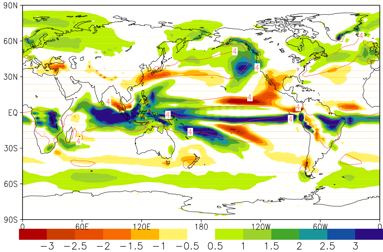
cmip5 ipsl rcp8.5 DJF Prec(2070-99) (1850-79)
