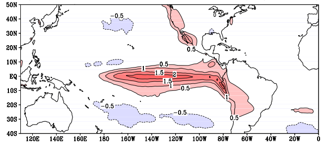
ENSO-Clim DJF: CNRM cmip5(amip) Ts (83 87 92 95 98 03) - (79-05clim)
