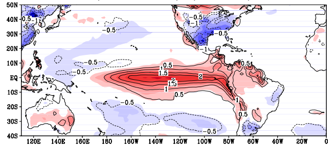
ENSO-Clim DJF: INMCM4 cmip5(amip) Ts (83 87 92 95 98 03) - (79-05clim)
