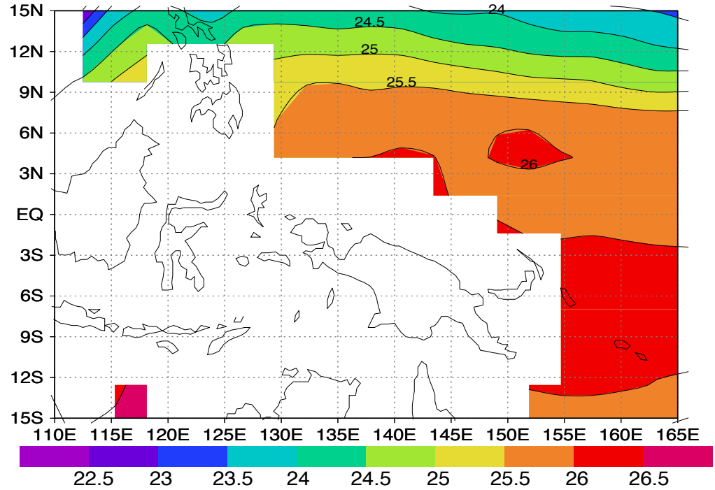
T 1000 ccsm3 DJF 0k
