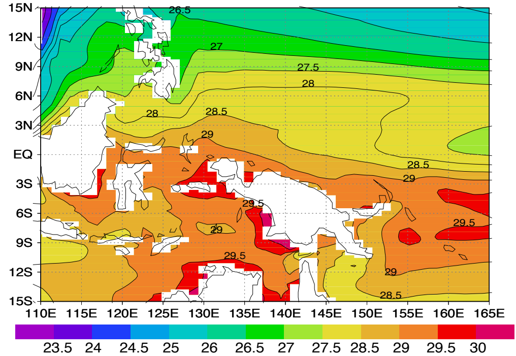
sst ccsm3 DJF 0k
