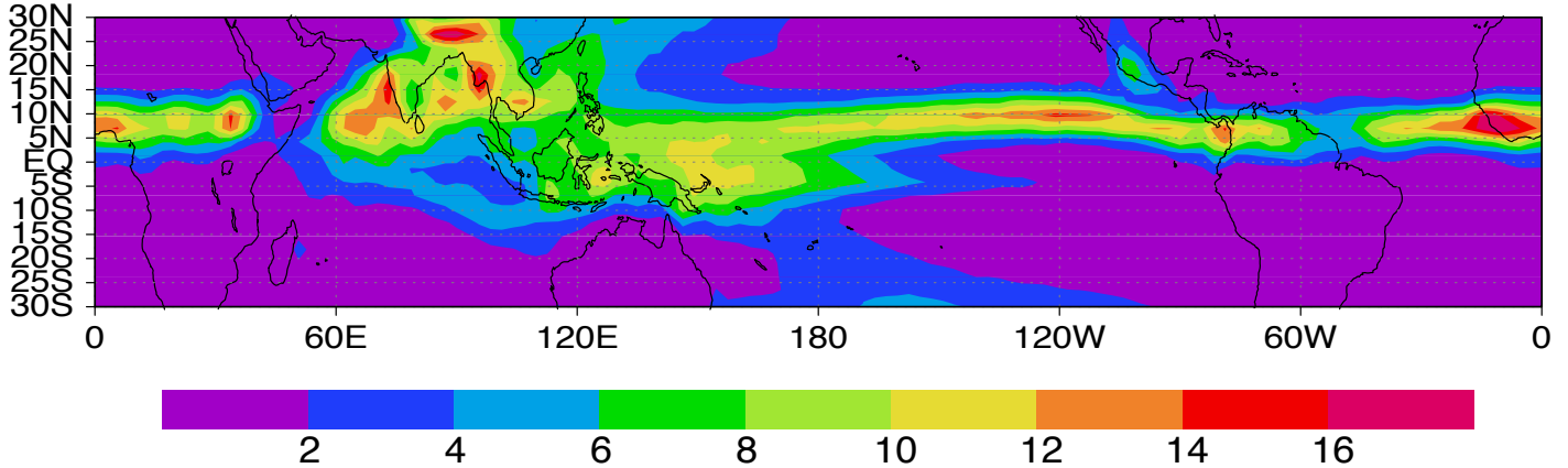
prec miroc JJA 0k
