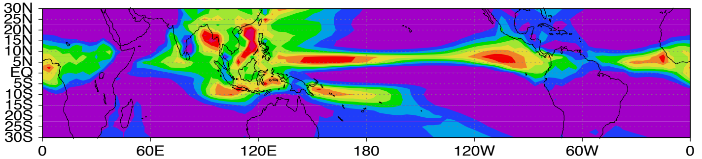
prec hadcm3m3 JJA 0k
