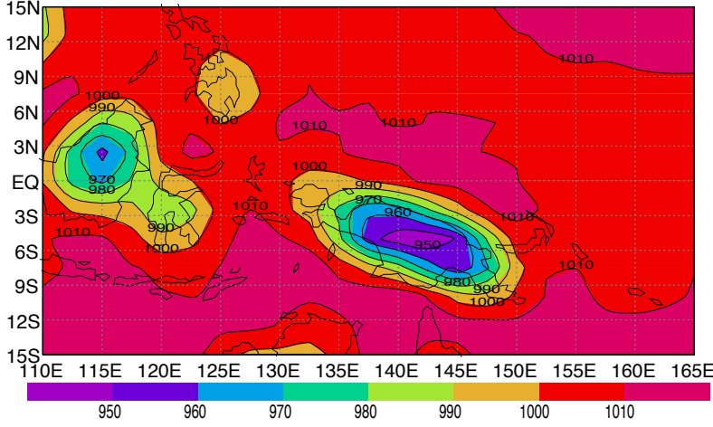
sfc pres ccsm3 JJA 0k
