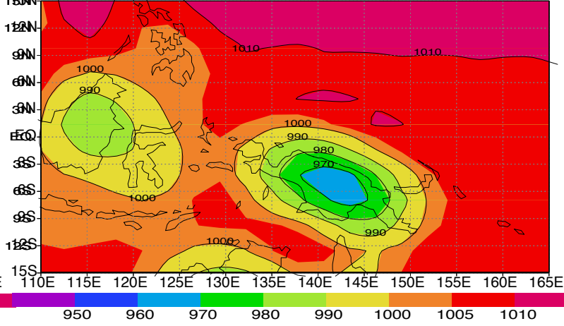
sfc pres haccm3m3 DJF 0k
