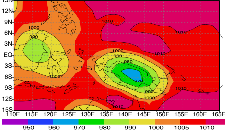
sfc pres haccm3m3 JJA 0k
