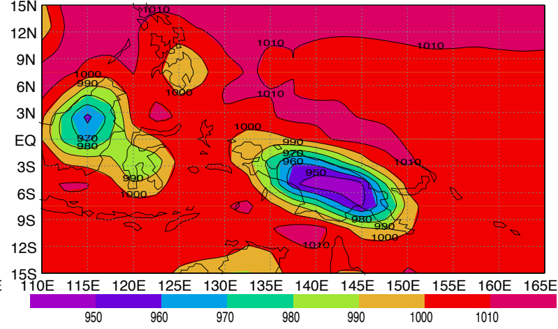
sfc pres ccsm3 DJF 0k
