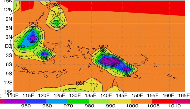
sfc pres miroc DJF 0k
