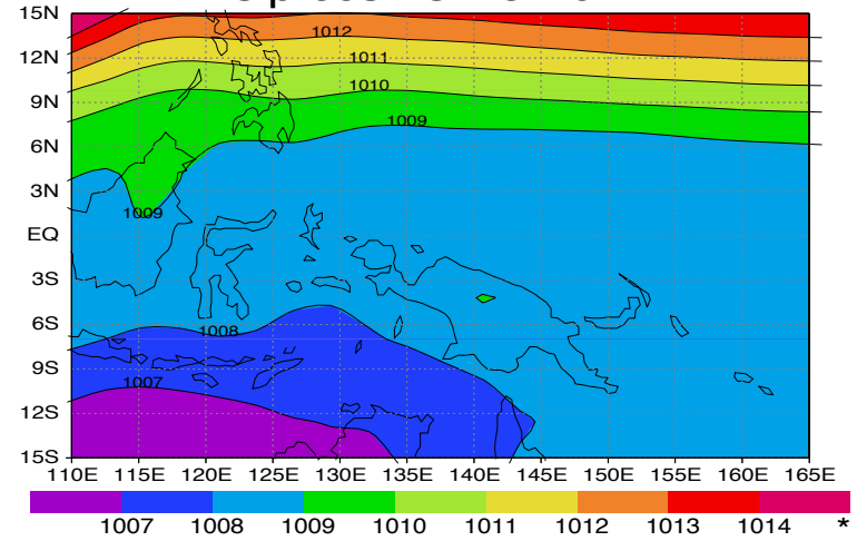
slp haccm3m3 DJF 0k
