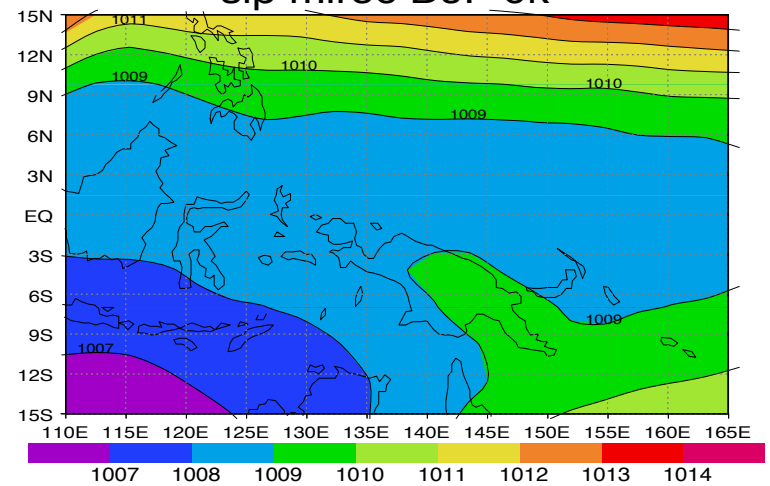
slp miroc DJF 0k
