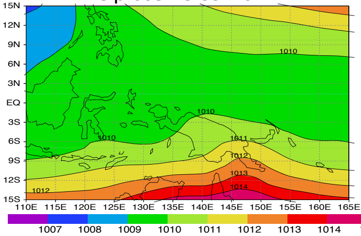
slp haccm3m3 JJA 0k
