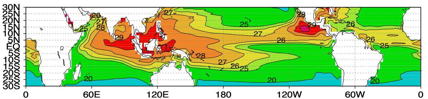
sst miroc JJA 0k
