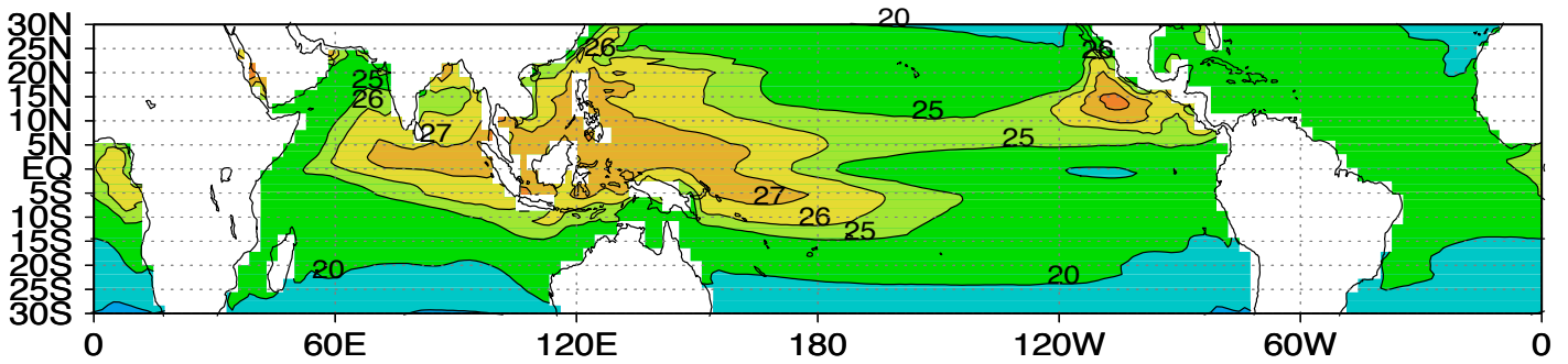
sst miroc JJA 21k
