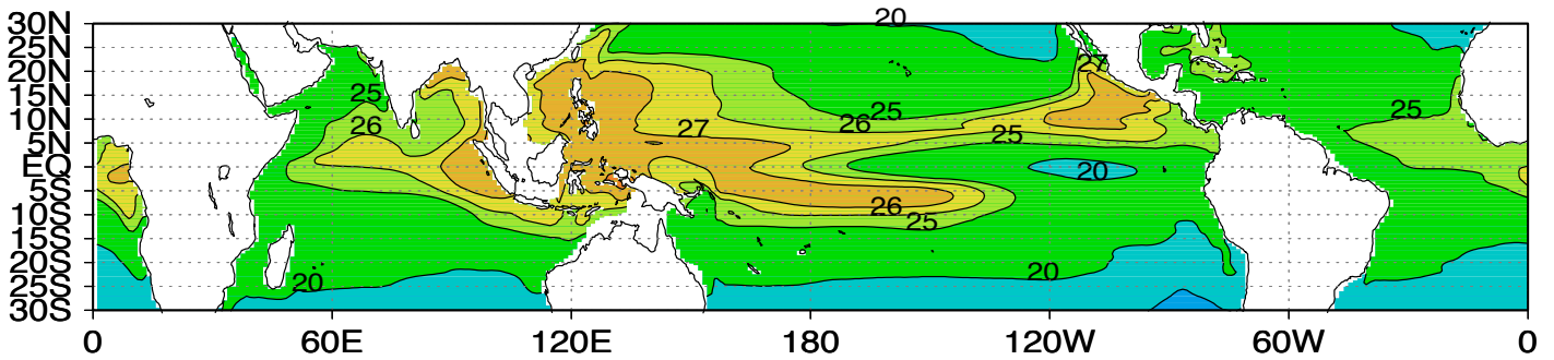
sst ccsm3 JJA 21k
