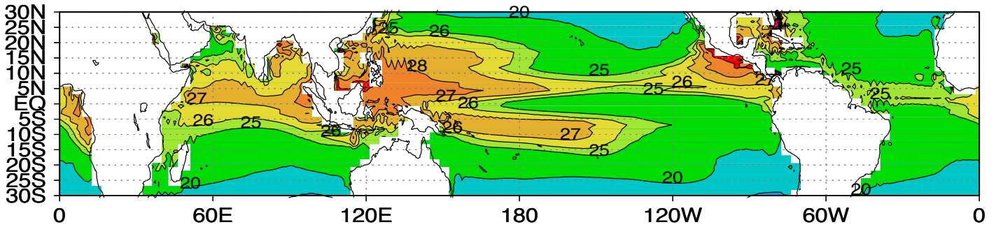
sst miroc JJA 21k
